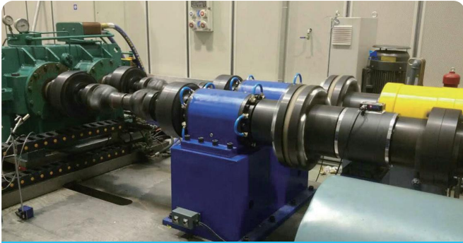
试验台系统
